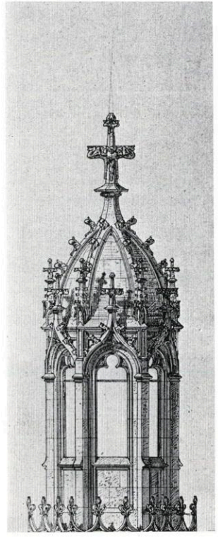
34. Entwurf für eine Umgestaltung des Eicheltürmchens von F. J. Denzinger (nicht ausgeführt), 1869.
